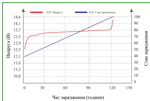
Крива розрядження при різних температурах (0,5C)
