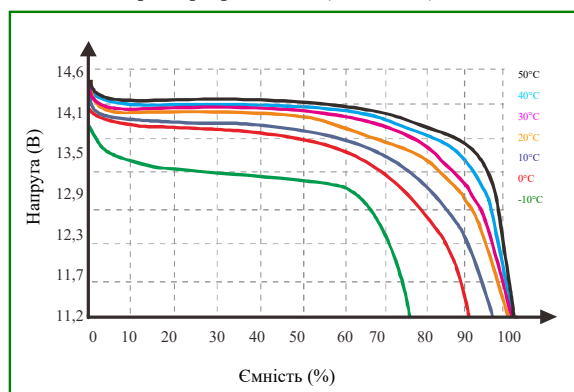
Крива розрядження (0,5C, 25°C)
