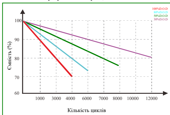
Кількість циклів в залежності від %DOD розрядження при 0,2C 25°C
