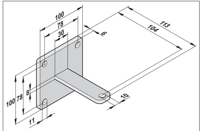
Кронштейн створки ворот (размеры в мм)
