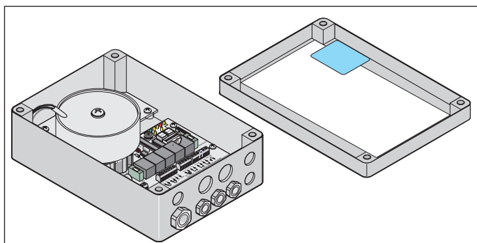
Рис. Система управления с заводской табличкой на внутренней стороне крышки
