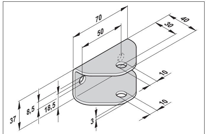
Кронштейн деревянной стойки ворот (размеры в мм)
