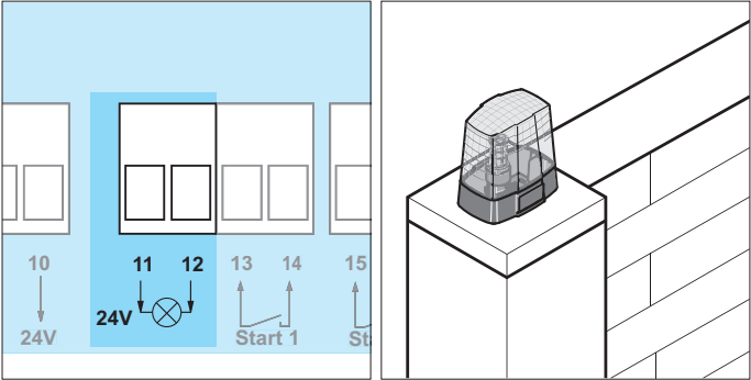
Рис. Соединительная клемма Рис. Предупреждающий световой сигнал 24 В
