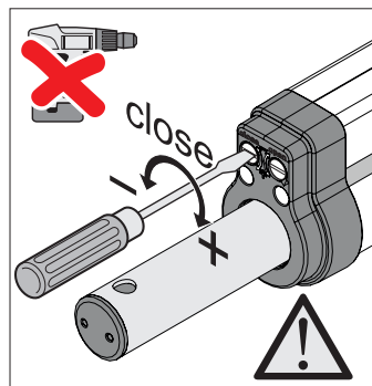
Рис. Направление вращения регулировочных винтов (close)
