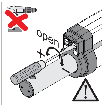
Рис. Направление вращения регулировочных винтов (open)
