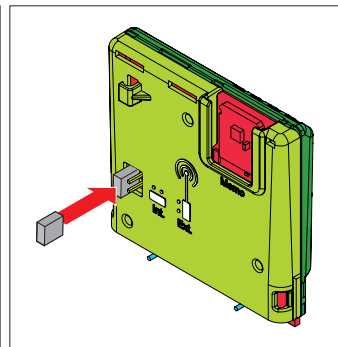
Рис. 2 Переключатель внешней антенны
