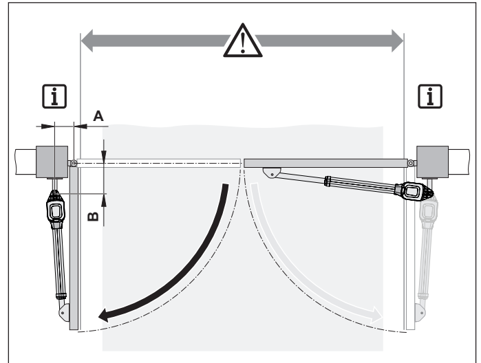
Рис. Открытие системы ворот вовнутрь
