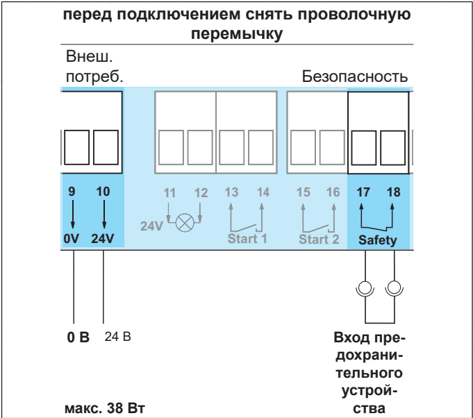
Рис. Соединительная клемма Рис. Предупреждающий световой сигнал 24 В
