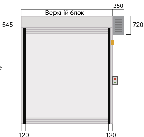
Фронтальний розріз
