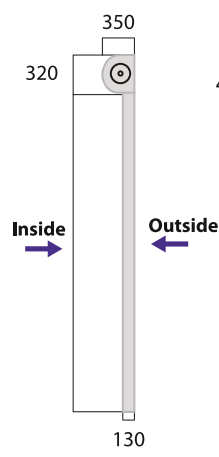
Поперечний розріз
