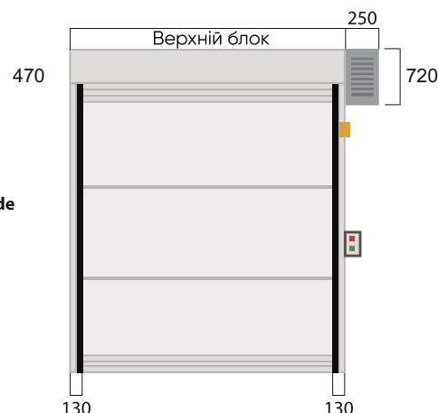
Фронтальний розріз
