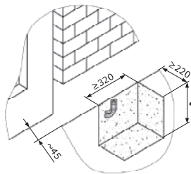
Малюнок 2. Підготовка під фундамент
