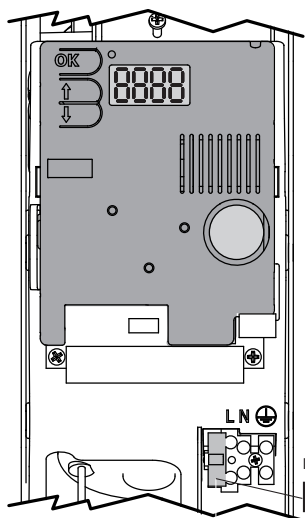
Плавкий предохранитель 1,6 AT
