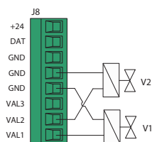
Рисунок 6. Подключение клапанов
