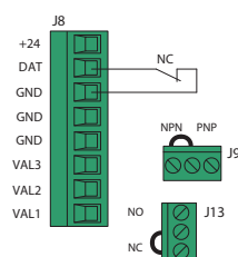
Рисунок 7. Подключение кнопок управления и светодиода (рис. 1)
