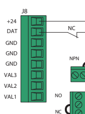
Рисунок 8. Подключение датчика положения ворот:
