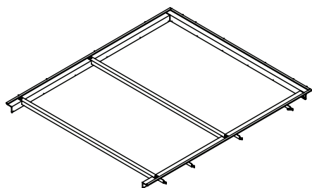
Предварительно устанавливаемая рама
